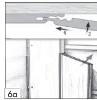
Mount the remaining panels. Weitere Paneele montieren.
