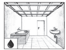
Batten frame – wet room Kantenlattung bei Feuchträumen
